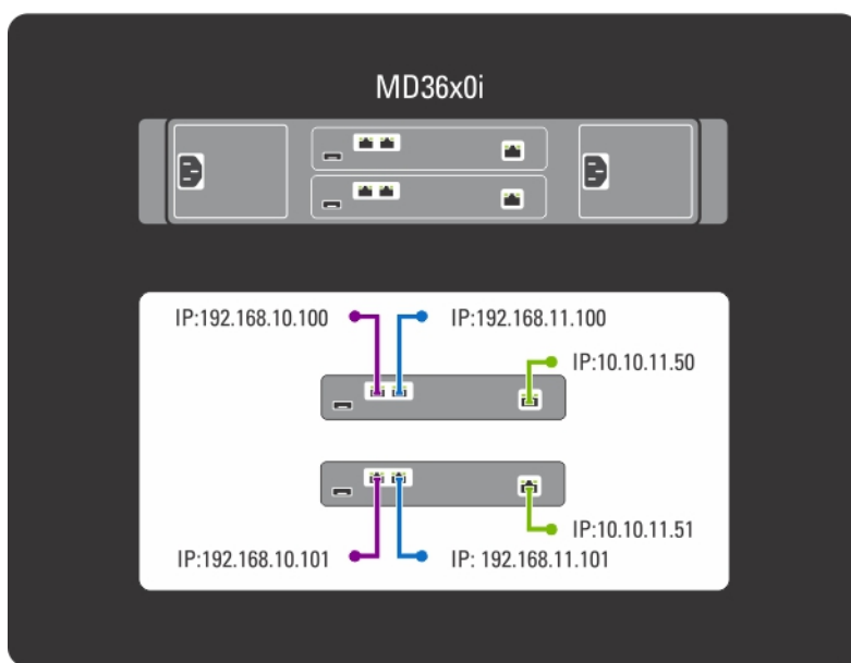
图 1: MD 交换机拓扑
