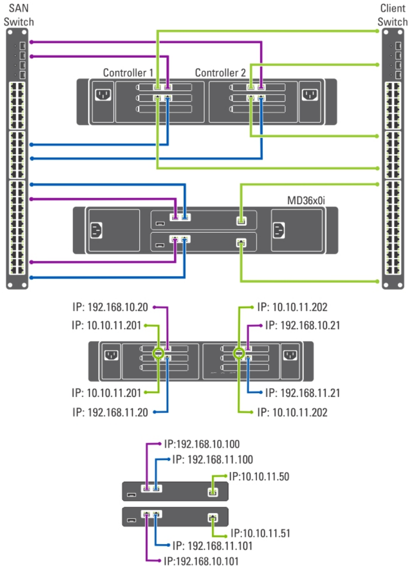
图 4: 非冗余选项中的专用 SAN 解决方案
