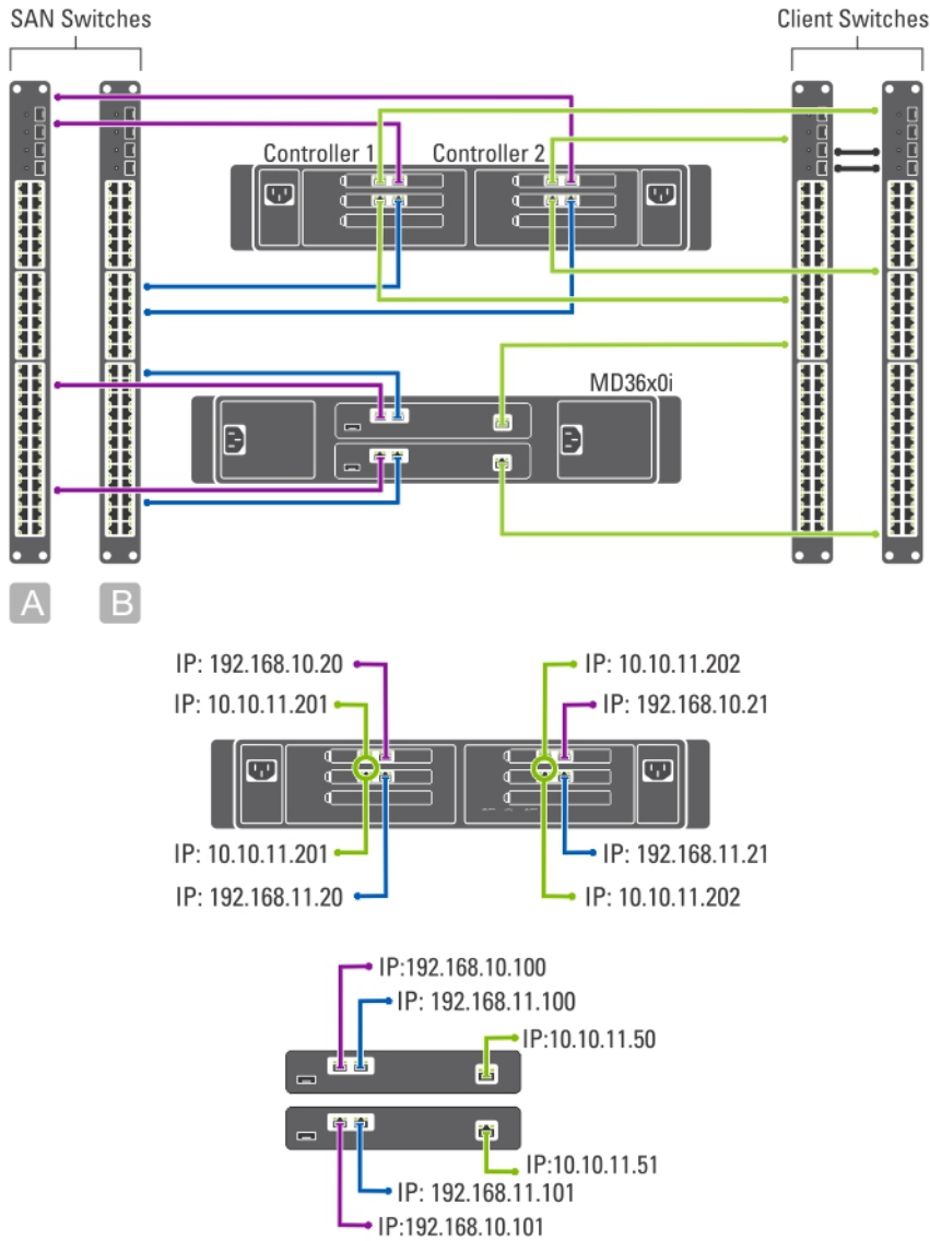
图 3: 高可用性选项中的专用 SAN 解决方案
